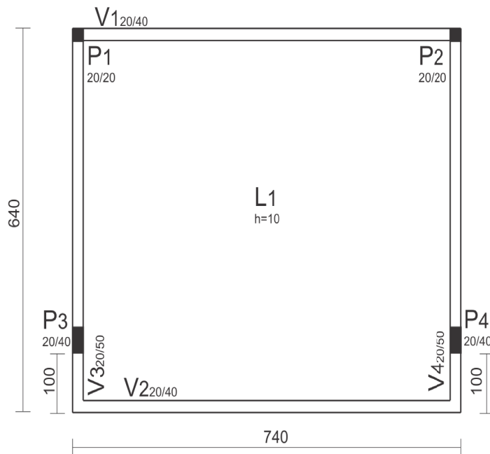
Figura 1 – Planta de fôrma (dimensões em cm)
