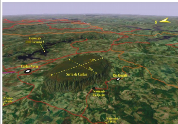
GOIÁS (Estado). Hidrogeologia do Estado de Goiás . 2006. 232p. p. 190. (Figura 12.2).
