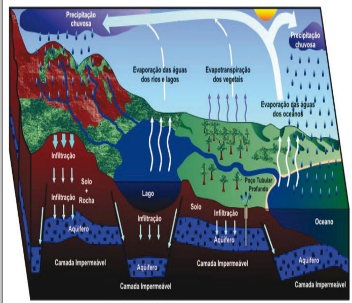
GOIÁS (Estado). Hidrogeologia do Estado de Goiás . 2006. 232p. p. 20. (Figura 1.3.)
